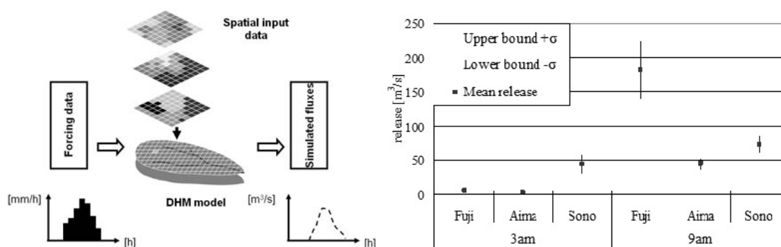
図 8 分布型水文モデルのスキーム(左)と各ダムにおける 6 時間ごとの適切放流スケジュールの例(右)
