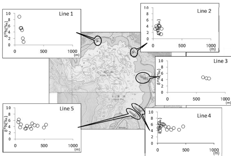
図 7 石垣島名蔵湾内に生息するリュウキュウスガモの安定同位体比の変化 (横軸:陸からの距離、縦軸:窒素安定同位体比)
