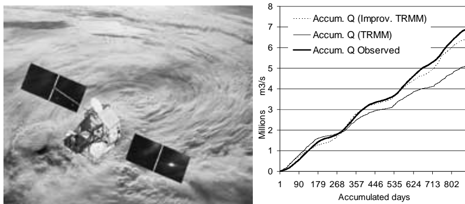
図9 TRMM 衛星降雨イメージ(左)と衛星データを活用した流量予測の改善例 (右、バングラディッシュ Bairab Bazar)
