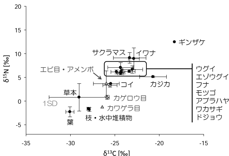
図 5 同位体比を用いた寒河江ダム貯水池における食物網の解明
