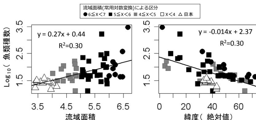
図 11 世界の代表的河川の流域面積及び緯度と魚類種数の関係 (左右とも有意な相関関係、 \alpha=0.05 )。
