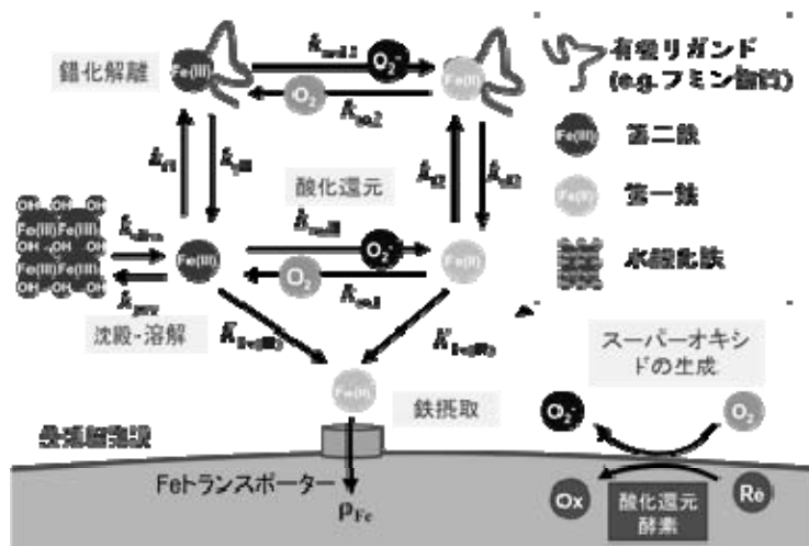
図 1 水中での鉄の化学反応と藻類による利用
