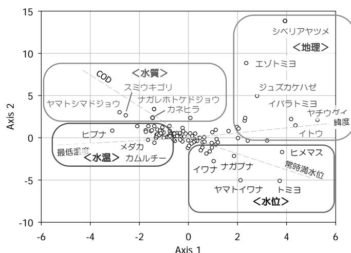
図 6 全国のダム貯水池を対象とした魚類群集と環境条件との対応(正準対応分析)
