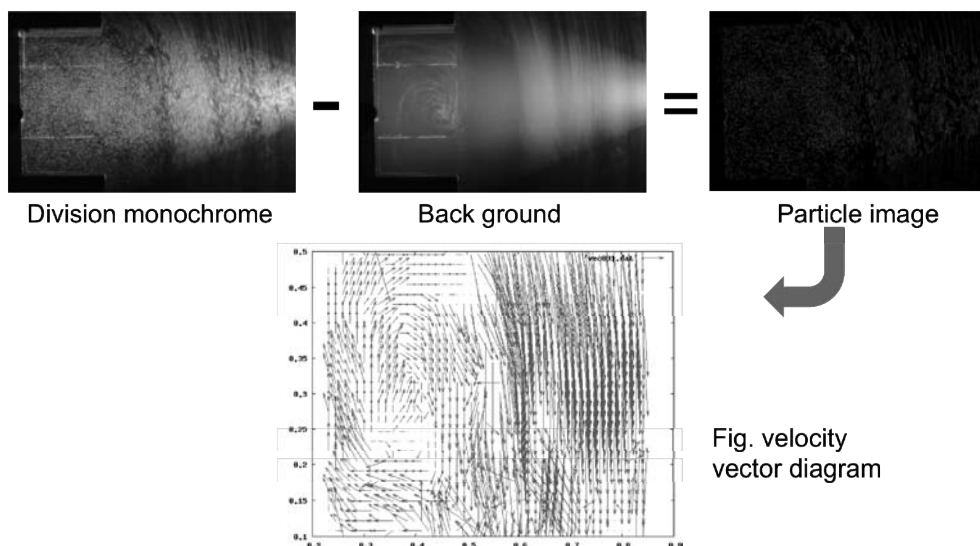
図2 水制を有する開水路での PIV 法による流速場の計測
